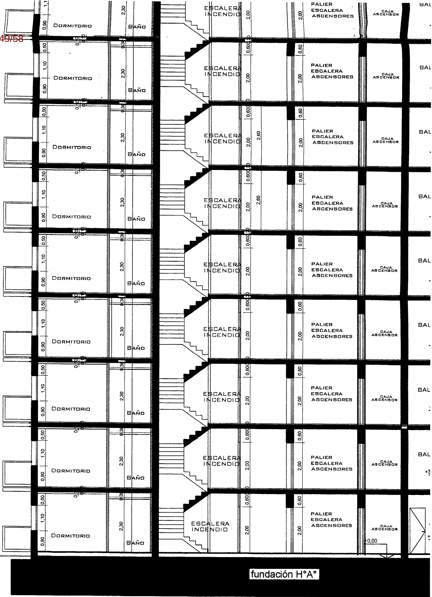
CORTE A-A ESC.: 1:100
