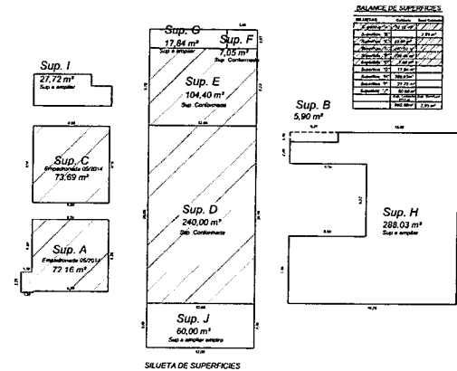
SILUETA DE SUPERFICIES Escala 1:200
