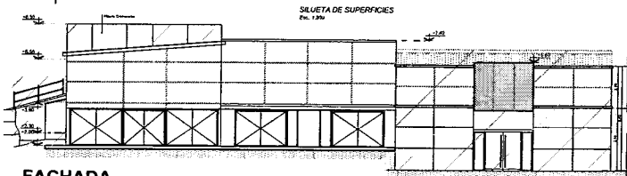
FACHADA ESCALA 1/100
